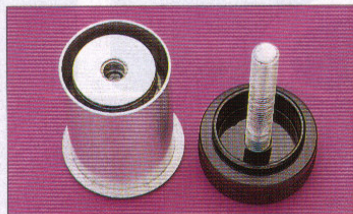
Vier solcher silikongefüllten Fertigtöpfe tragen das Subchassis. Sie werden von Gewindestangen mit schwarzen Kunststoffkappen gekontert
